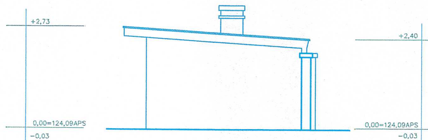
ZAPADNO PROCELJE
