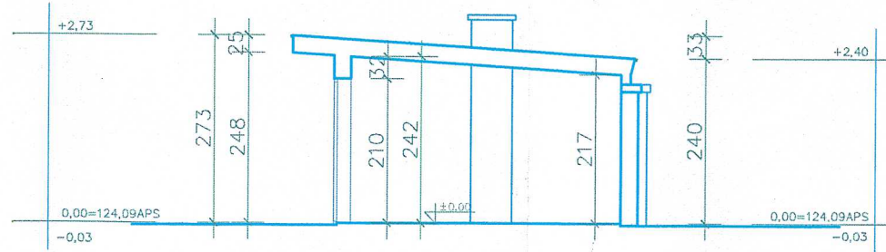
PRESJEK A-A
